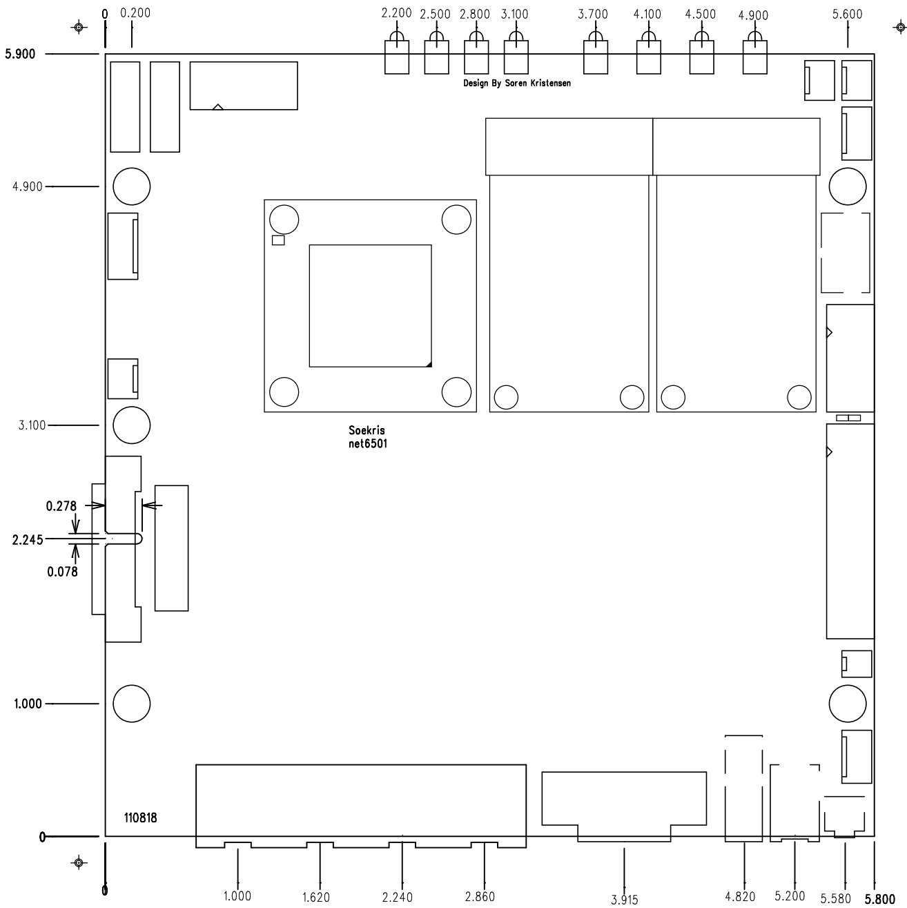
Layer 1 (Top)
